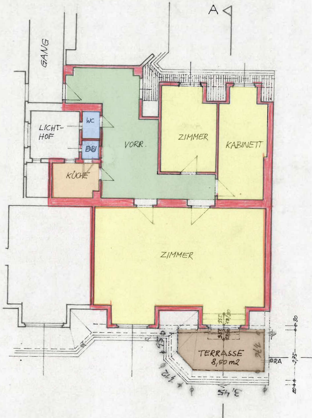
GRUNDRISS 1:100
