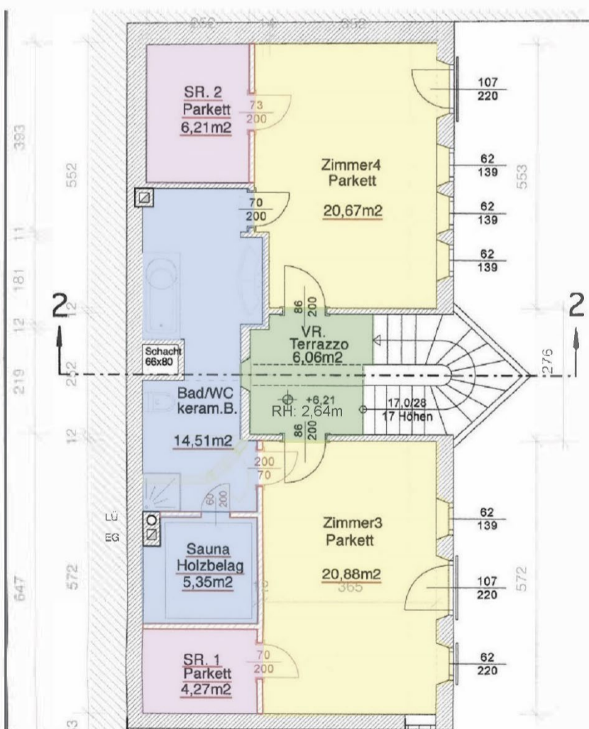
2. OBERGESCHOSS
