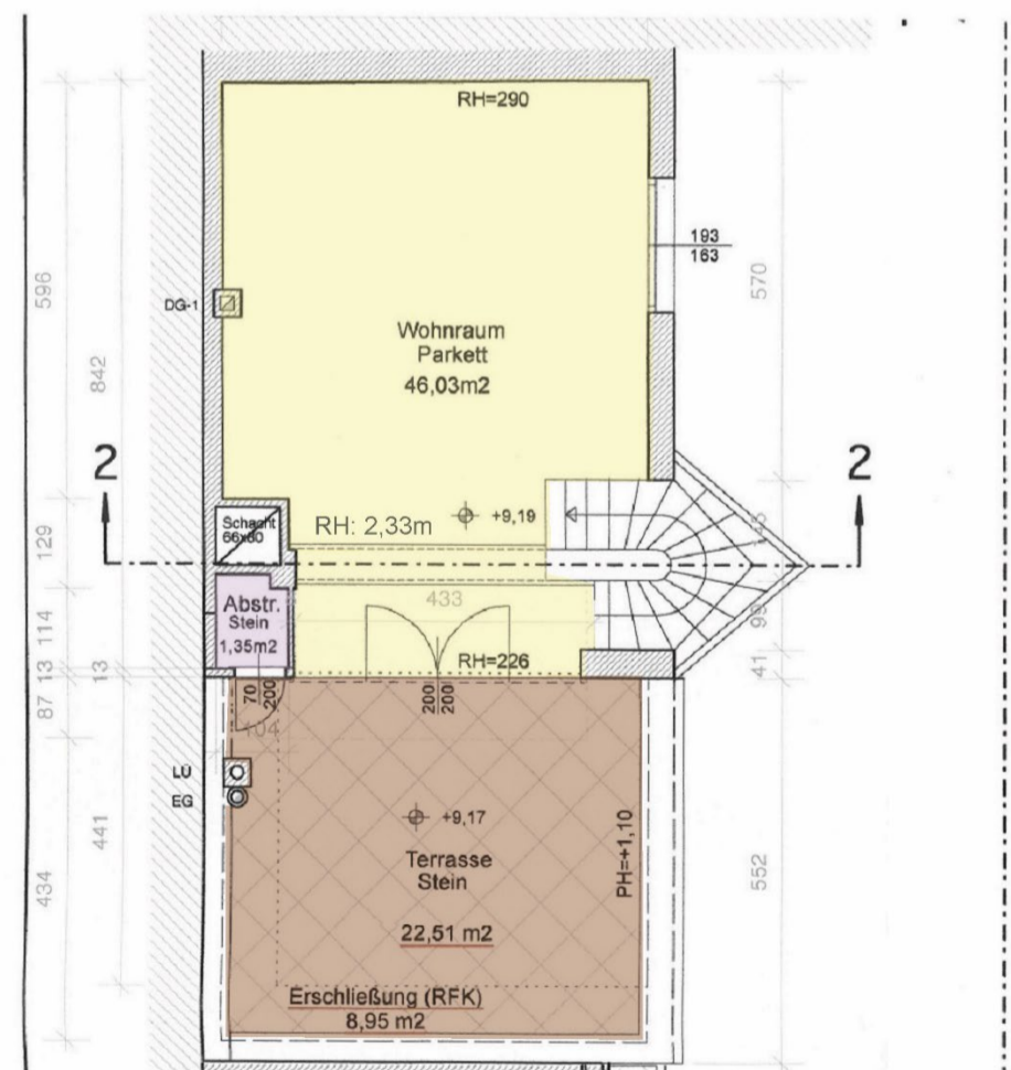
1. DACHGESCHOSS
