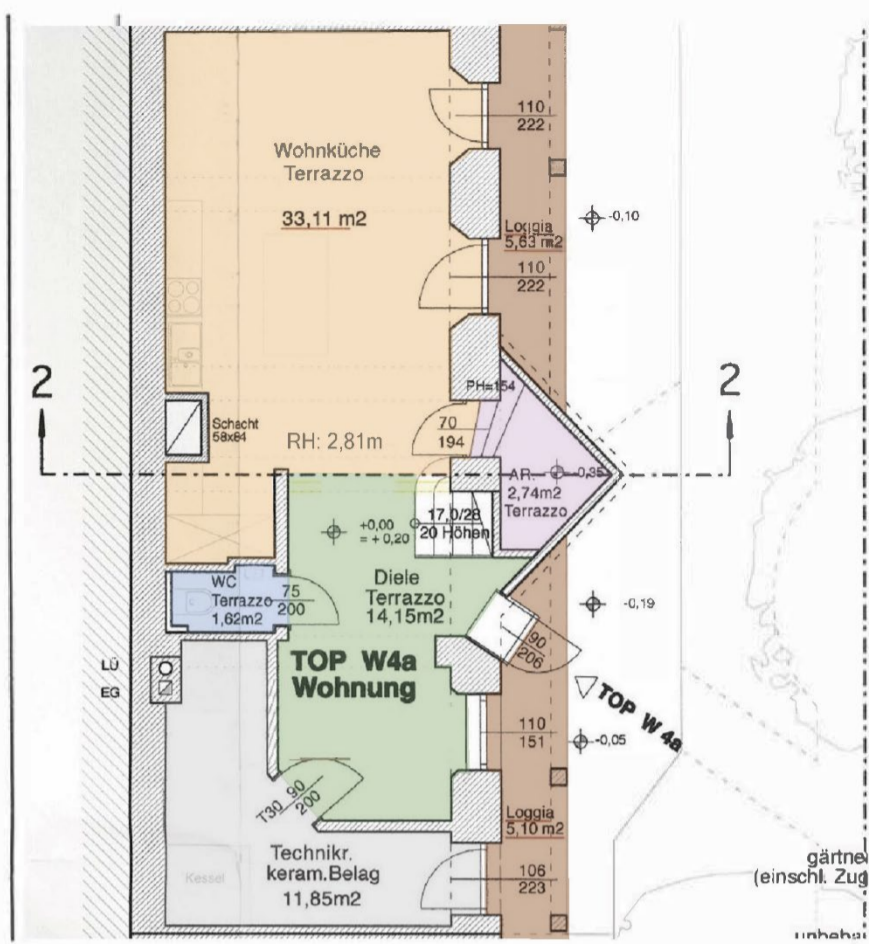
ERDGESCHOSS
